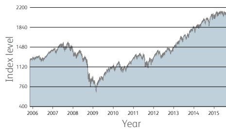
S&P 500 Index
